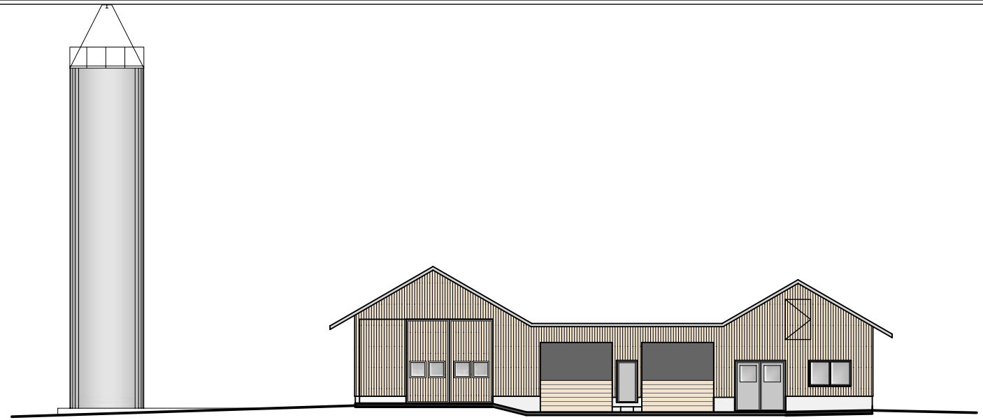
Südfassade
