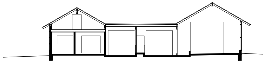
Schnitt A--A
